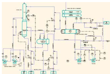
MEDUSA4 P&ID permet de traiter facilement les diagrammes complexes
